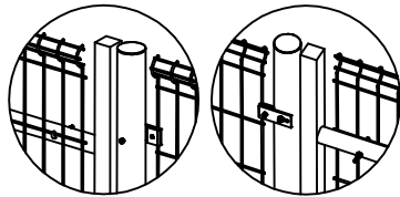
ロッカー用部材&J型ボルト取り付け
