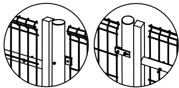
ノッカー用部材&J型ボルト取り付け
